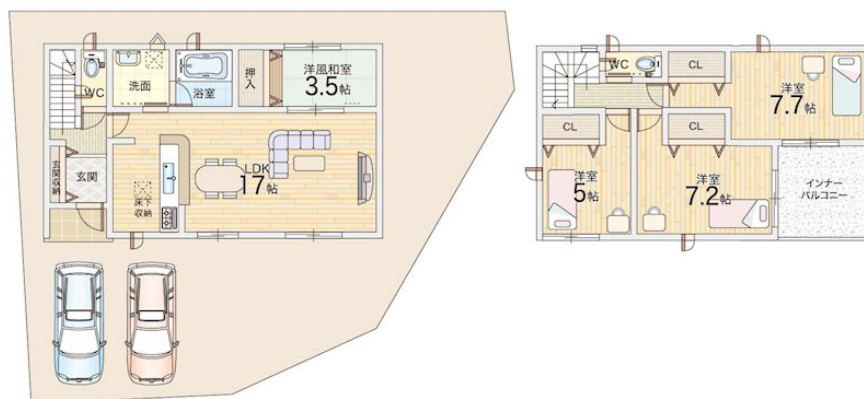
【間取り図】
