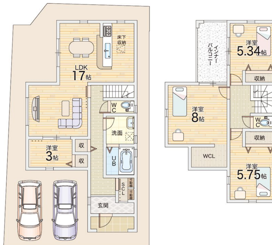
【間取り図】
