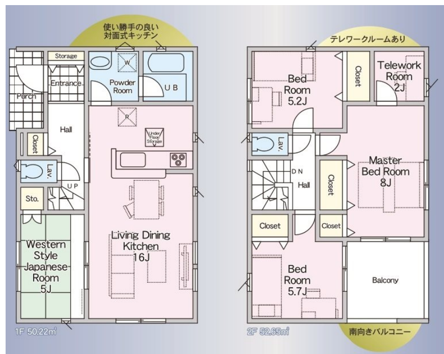
【間取り図】
