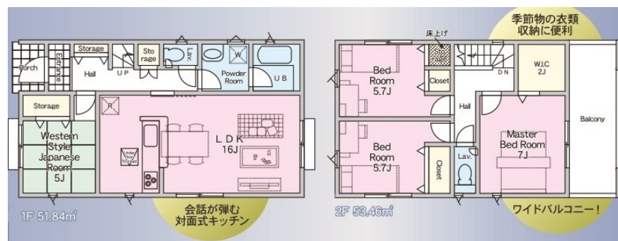
【間取り図】
