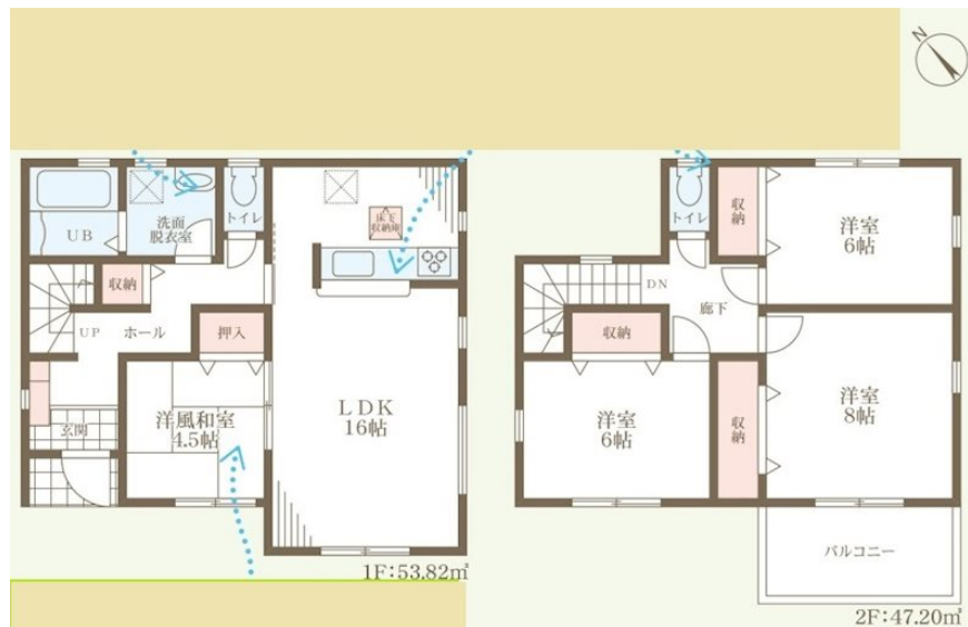
【間取り図】
