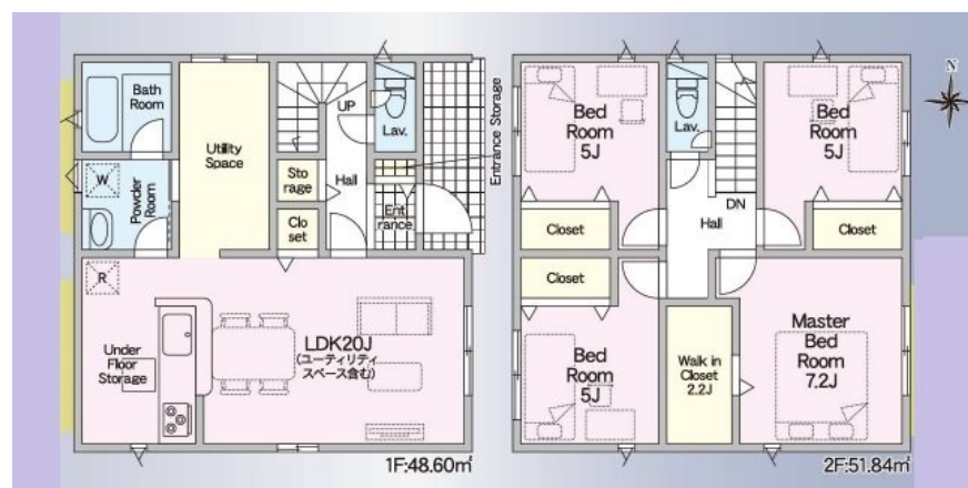
【間取り図】
