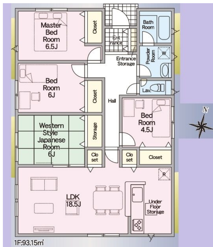
【間取り図】
