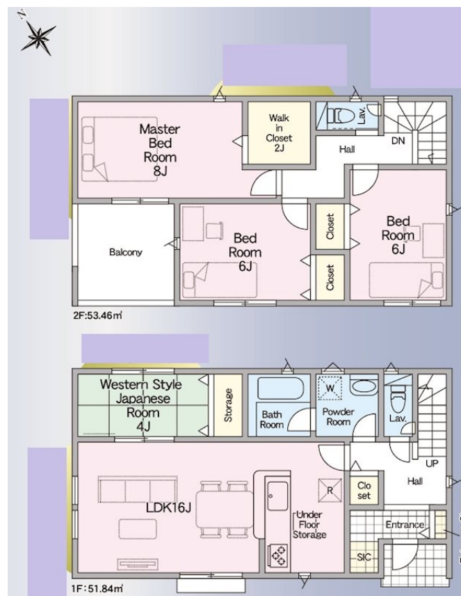
【間取り図】
