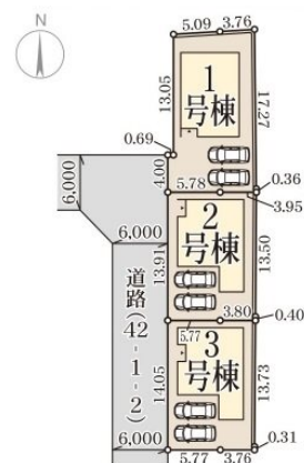
区画図
